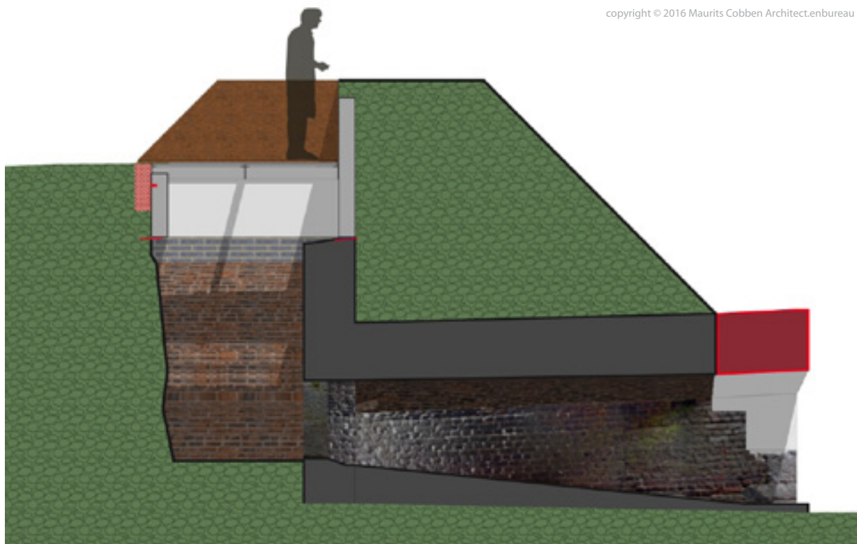
doorsnede over geschutstrechter en kazemat met afdekking van beloopbaar glas
