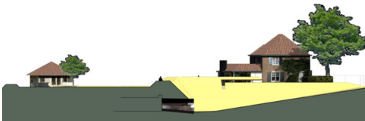
doorsnede over uitgegraven schootsveld geschutstrechter
